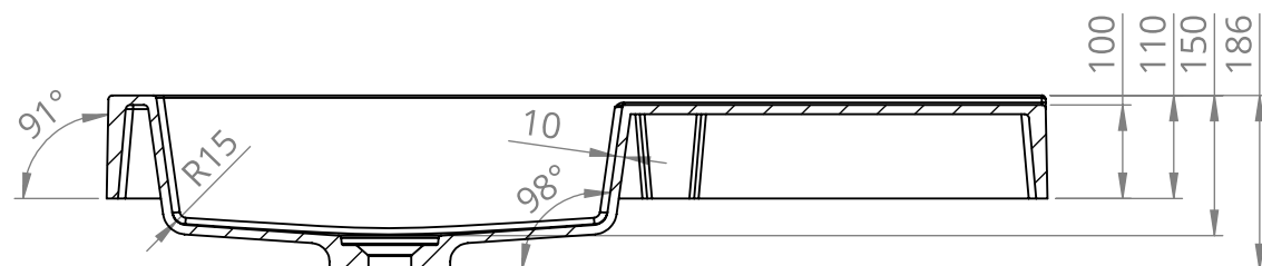
PRZEKRÓJ H-H SKALA 1 : 9
